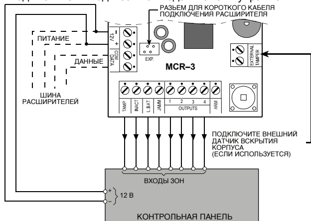
Рисунок 5. Схема подключения
